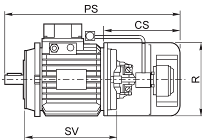
Ventilazione forzata con encoder e freno Forced cooling with encoder and brake Zwangsbelüftung mit Encoder und Bremse
